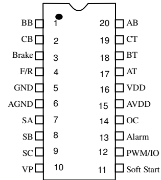
L33035A/B (SSOP20)
